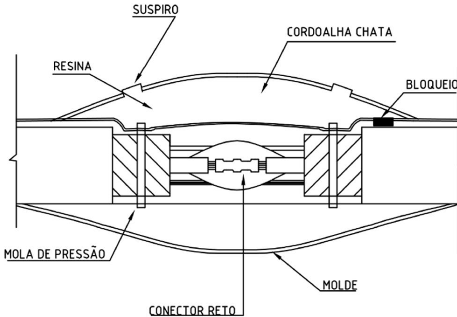
Figura 1 - Emenda reta para cabo de potência tetrapolar com armação 0,6/1,0 kV
